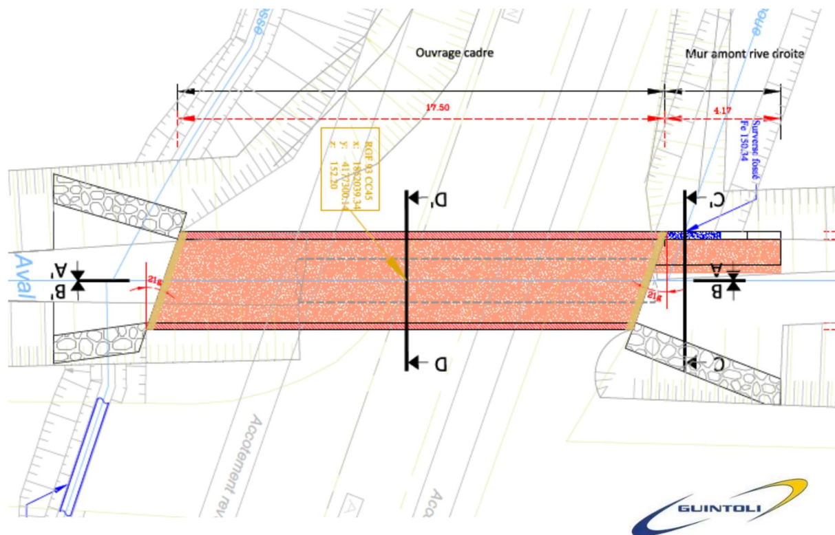
Positionnement du moule sur les armatures
